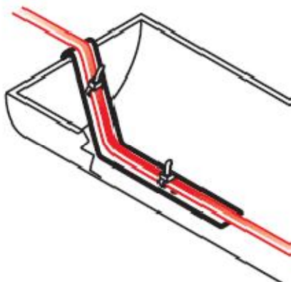
Переход в водосточный желоб.
