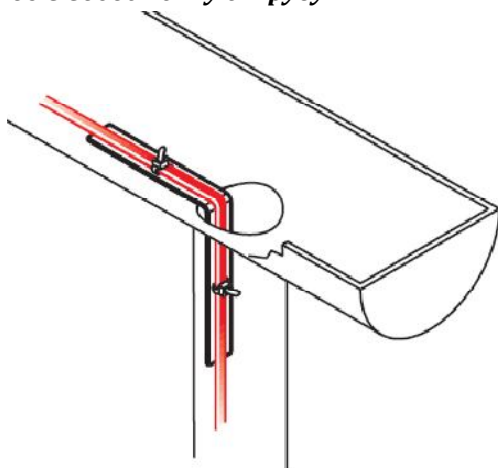
Переход в водосточную трубу.
