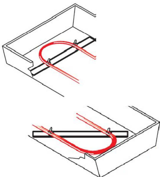
Фиксирование расстояния между нагревательными нитками
