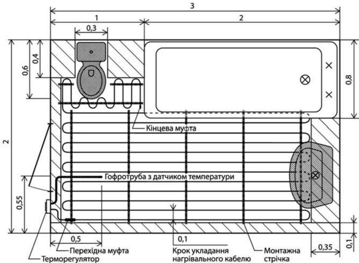
Рисунок А.3 - Розташування елементів ЕКС ТП
