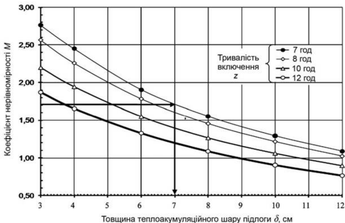
Рисунок 1 - Залежність товщини теплоаккумуляційного шару підлоги від коефіцієнта нерівномірності M при різних тривалостях включення ЕКС ОТА
